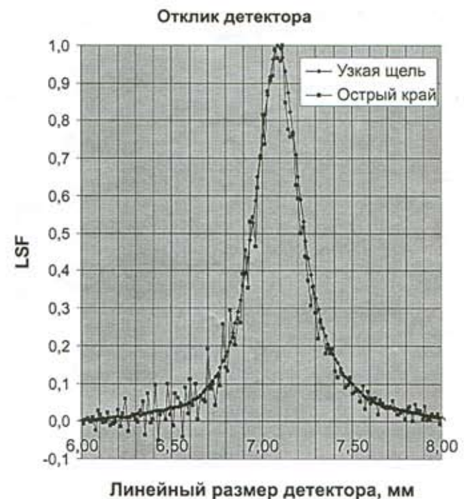
Рис. 4. Отклик детектора на тест-объекты «острый край» и «узкая щель»
