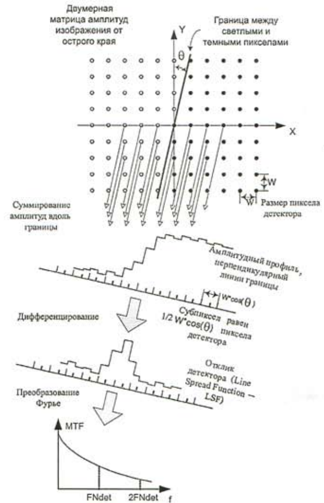
Рис. 2. Схема алгоритма субпиксельной угловой проекции
