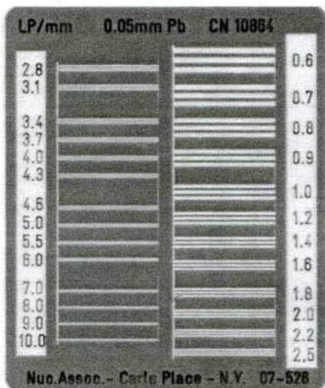
Рис. 5. Тест-объект разрешения «штриховая мира»
